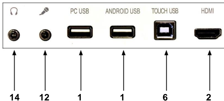
Přední panel
